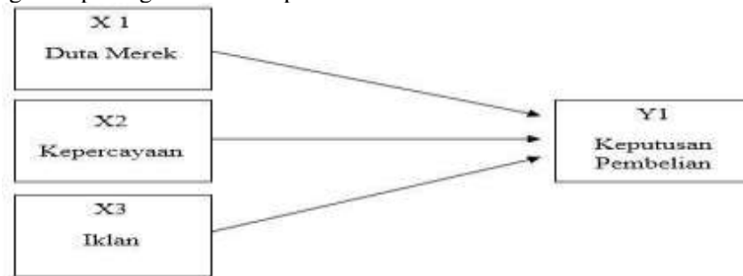
Gambar 4. Kerangka Berpikir
