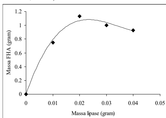
Gambar 3. Pengaruh jumlah massa lipase terhadap pembentukan FHA
