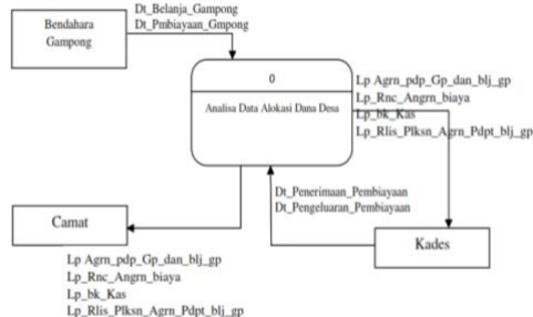
Gambar 2. Diagram konteks sistem rancangan
