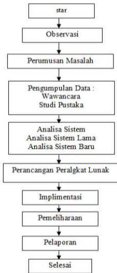
Gambar 1. Tahapan Penelitian
