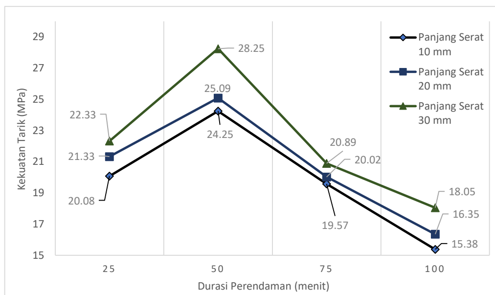
Gambar 5. Interaksi Panjang serat dan Durasi Perendaman.
