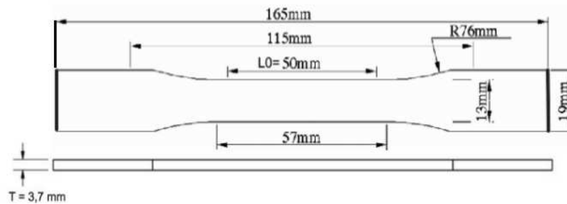
Gambar 2. Spesimen Uji Tarik.
