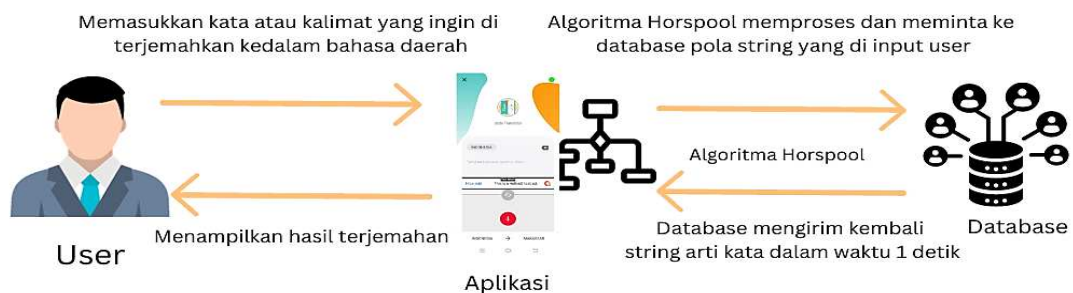
Gambar 1. Analisis Sistem
