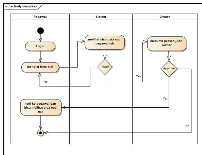
Gambar 7. Analisa Sistem Yang Digunakan
