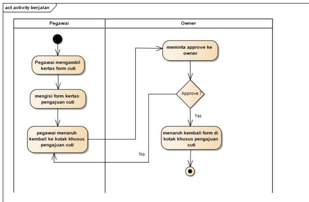
Gambar 6. Analisa Sistem Yang Berjalan
