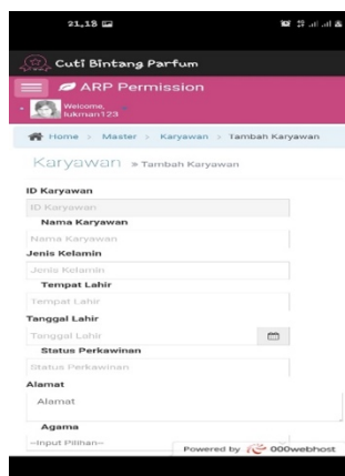
Gambar 3. Halaman Owner Untuk Input Pegawai Baru
