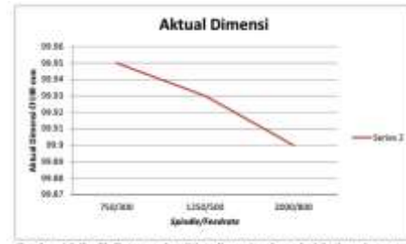
Gambar 4.6 Grafik Rata-rata ketelitian dimensi pada variasi feedrate dengan rpm yang berbeda
