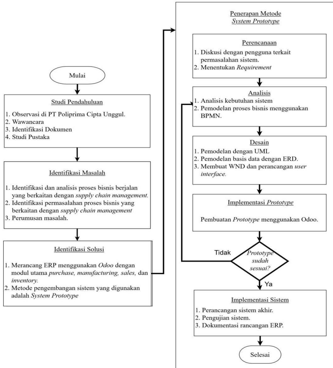
Gambar 1. Tahapan Penelitian
