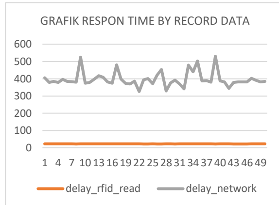
Gambar 4 Grafik respon time dengan pencatatan record data
