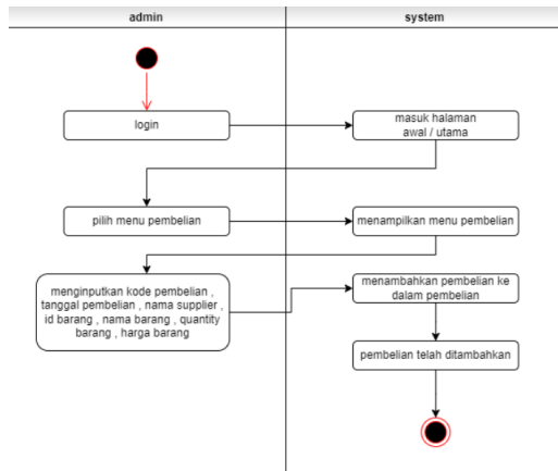
Gambar 3.12 Activity Diagram Pengeluaran Barang
