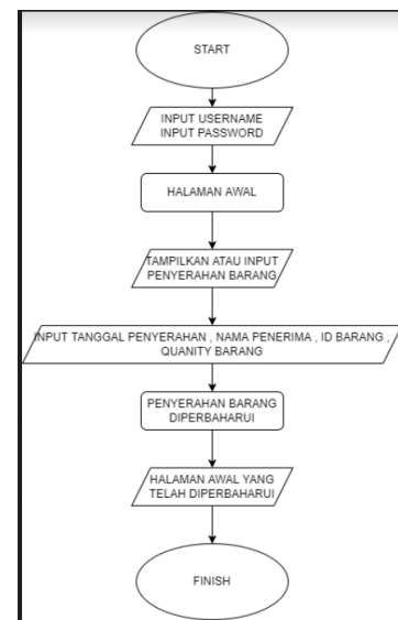
Gambar 3. 5 Flowchart Pengeluaran Barang
