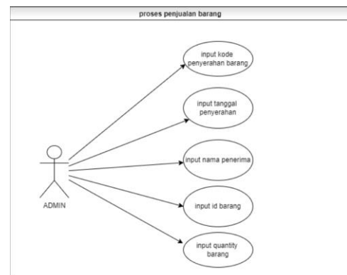
Gambar 3. 8 Use Case Pengeluaran Barang
