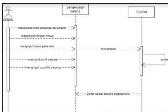
Gambar 3. 16 Diagram Sequence Pengeluaran Barang
