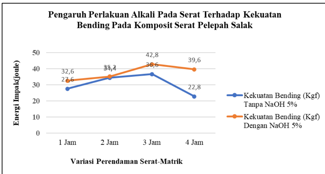
Gambar 9 Uji bending dengan perlakuan alkali serat salak dengan variasi perendaman 1 jam sampai dengan 4 jam.
