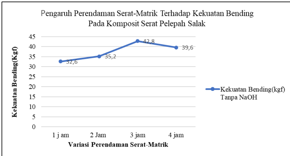
Gambar 8 Uji bending tanpa perlakuan alkali serat salak dengan variasi perendaman 1 jam sampai dengan 4 jam.
