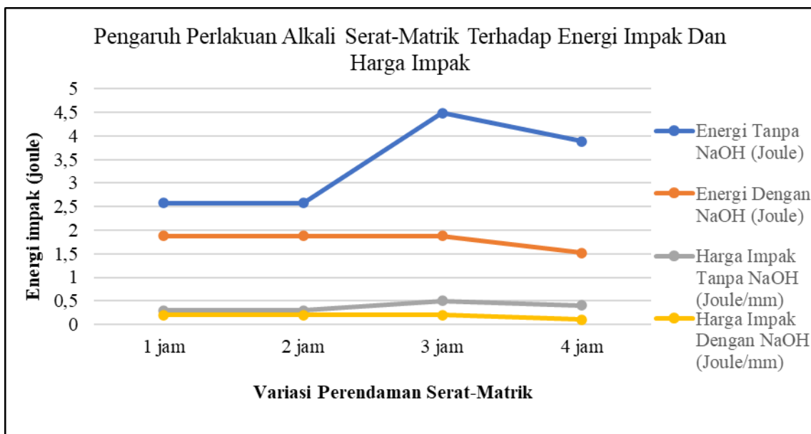
Gambar 7 Uji impact dengan perlakuan alkali serat salak dengan variasi perendaman 1 jam sampai dengan 4 jam.
