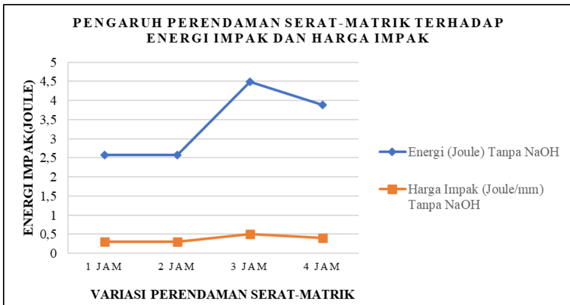
Gambar 6 Grafik uji impact tanpa perlakuan alkali serat salak dengan variasi perendaman 1 jam sampai dengan 4 jam.
