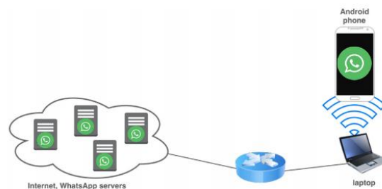
Gambar 2. Metodologi WhatsApp Forensics Dengan Internet Protocol (Marshall, 2008)
