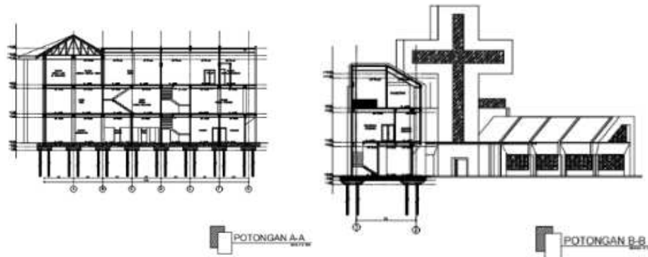
Gambar 11 : Potongan Sumber : analisa penulis
