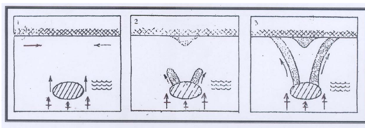
Gambar 4. Tombolo jenis ganda (Komar, 1975).
