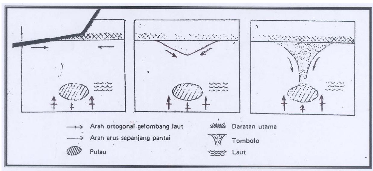
Gambar 3. Tombolo akibat lee side gelombang datang (Komar, 1975)
