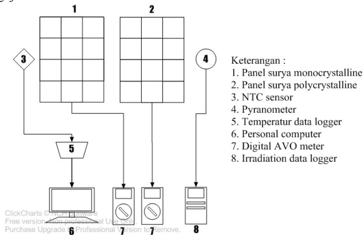
Gambar 1. Skema pengujian
