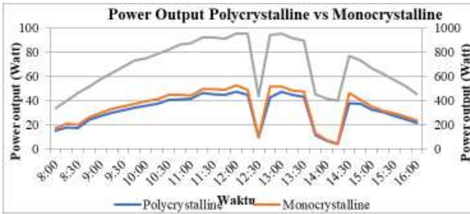
Gambar 3. Grafik daya panel surya dan intensitas radiasi matahari hari ke-1
