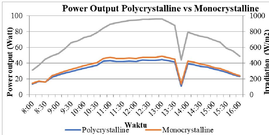
Gambar 4. Grafik daya panel surya dan intensitas radiasi matahari hari ke-2
