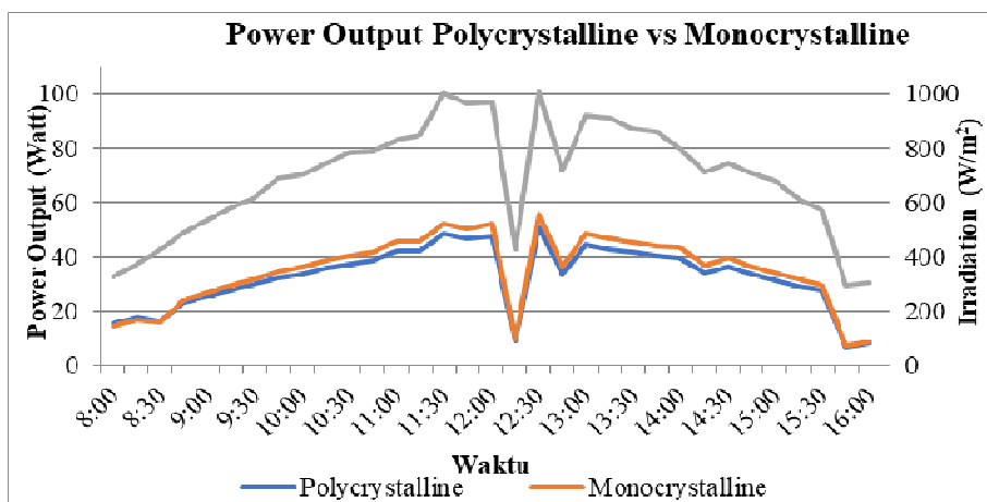
Gambar 5. Grafik daya panel surya dan intensitas radiasi matahari hari ke-3
