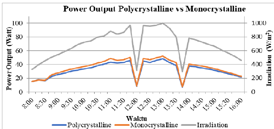
Gambar 6. Grafik daya panel surya dan intensitas radiasi matahari hari ke-4
