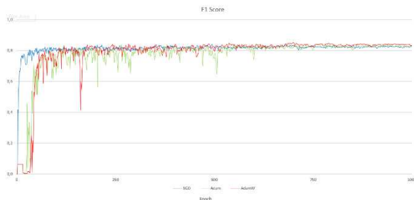
Gambar 8. Grafik kenaikan F1-score optimizer SGD, Adam, AdamW dalam 1000 epoch epoch
