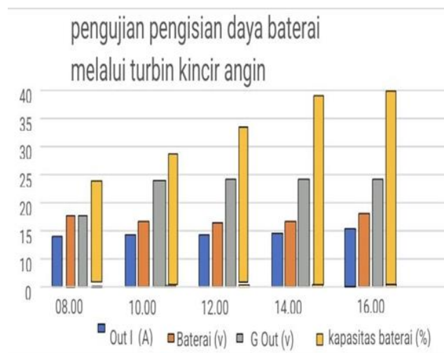
Gambar 13. Grafik pengujian pengisian daya baterai melalui turbin kincir angin Vertikal
