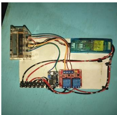
Gambar 8. Rangkaian pzem 004T
