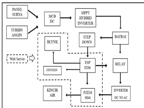
Gambar 1. Blok Sistem
