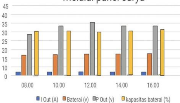
Gambar 12. Grafik pengujian pengisian daya baterai melalui panel surya
