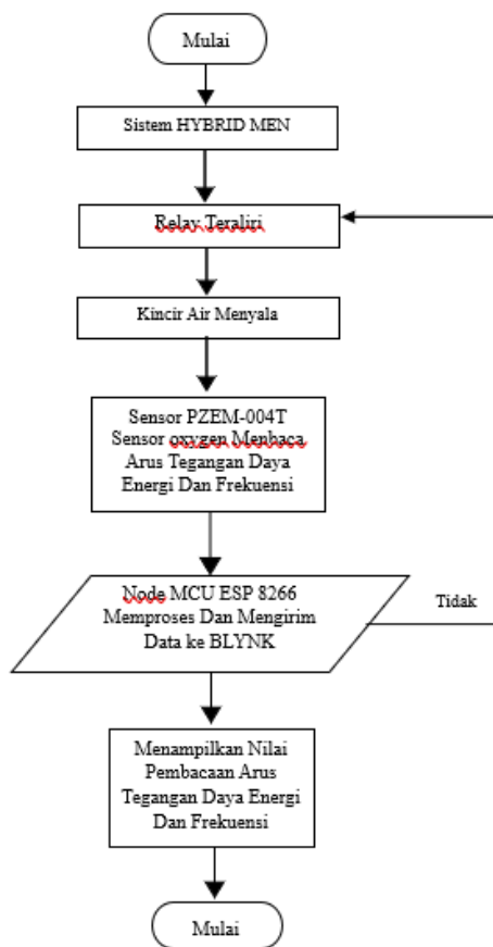
Gambar 3. Flowchart Sistem Kerja
