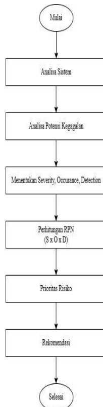
Gambar 1. Metodologi Penelitian
