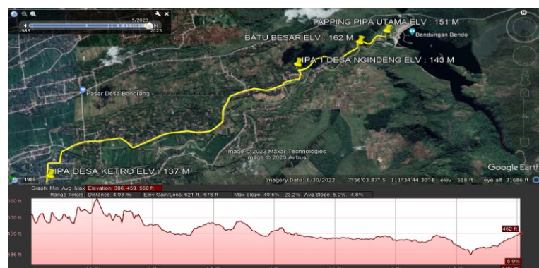
Gambar 2 Peta Long Section Jaringan Pipa Transmisi Bendo
