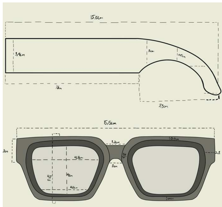
Gambar 4. Sketsa Ukuran Konsep Desain Awal (Sumber: Doc.Gallery.2024)
