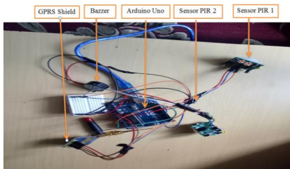
Gambar 8. Rancangan Hardware alat pendeteksi
