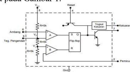
Gambar 1. Blok Dasar Ferwaktuan 555
