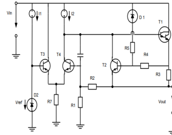
Gambar 3. Prinsip Rangkaian Ic 78xx
