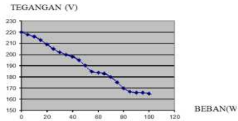
Gambar 4. Grafik Pengaruh Beban Terhadap Tegangan (V)
