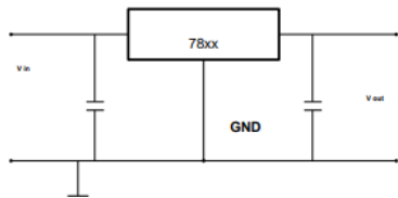
Gambar 2. Regulator Voltase Memakai Ic 78xx
