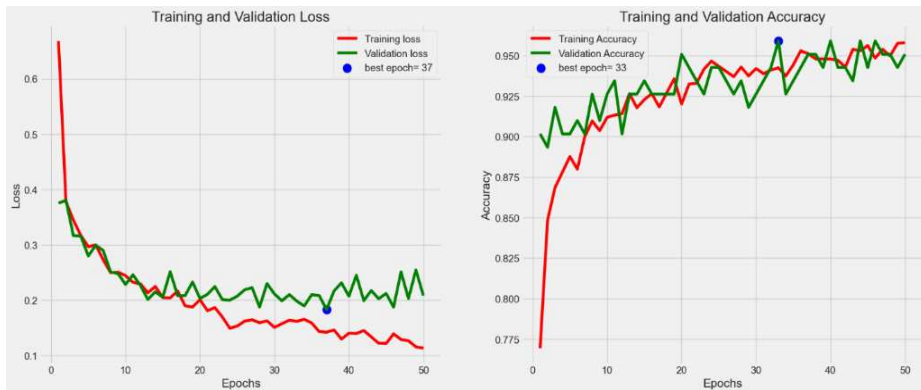
Gambar 5. Grafik Accuracy dan Loss pada VGG16 menggunakan augmentasi data
