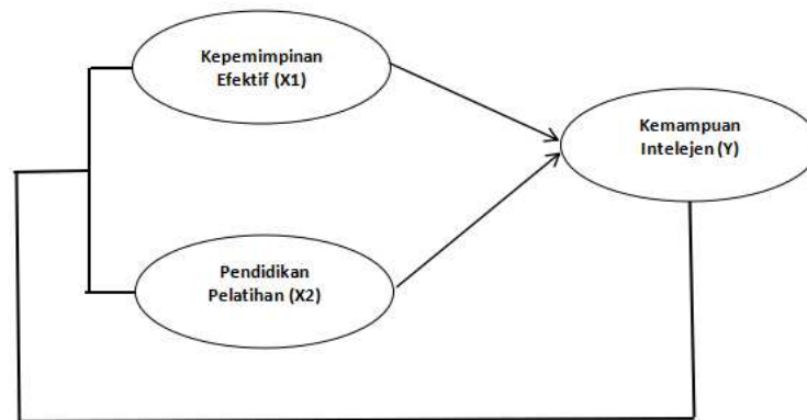
Gambar 1. Kerangka Konseptual
