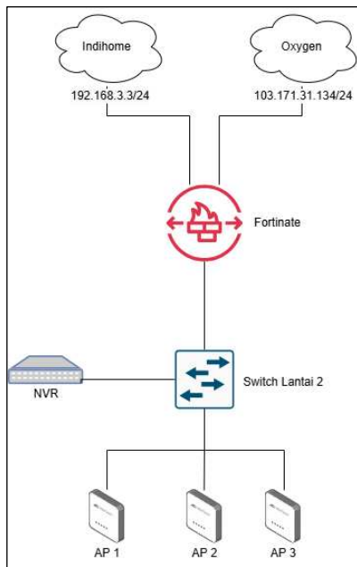
Gambar 4. Topologi Jaringan
