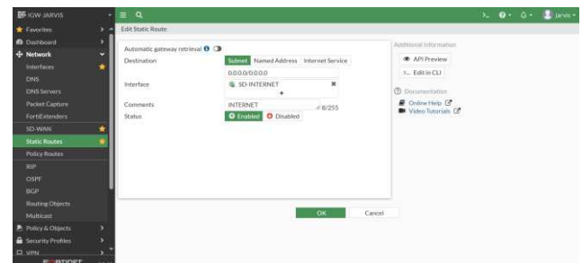
Gambar 7. Konfigurasi Static Route
