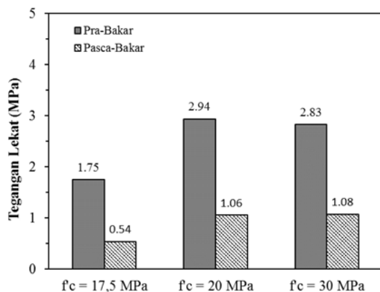
Gambar 9. Grafik Tegangan Lekat
