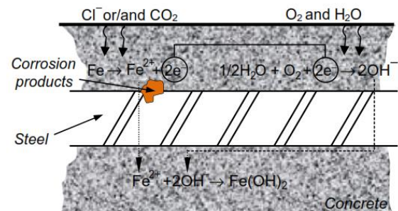
Gambar 2. Skema Ilustrasi Korosi Tulangan Baja pada Beton [1]
