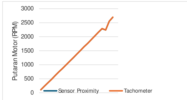
Gambar 8. Grafik Perbandingan Sensor Proximity dan Tachometer
