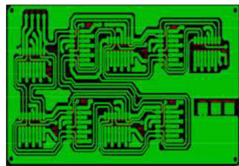
Gambar 6 Perancangan Print Layout PCB untuk Encoder Seven Segment
