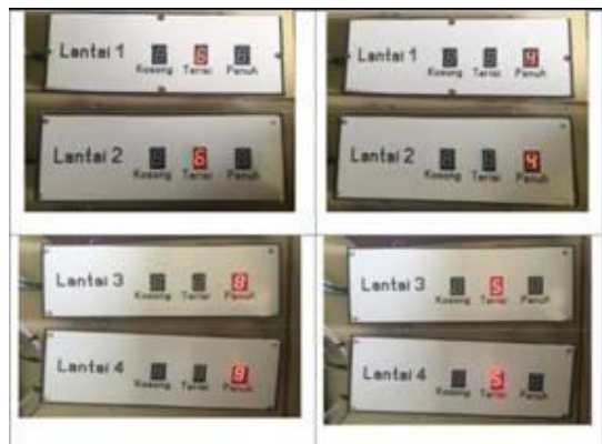
Gambar 11 Hasil Pengujian Sistem Scanning Pada Display Perlantai
