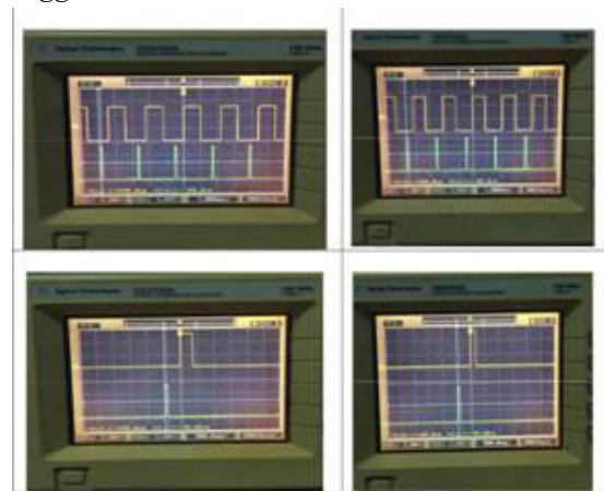
Gambar 14 Hasil Pengukuran Sinyal Echo dan Trigger
