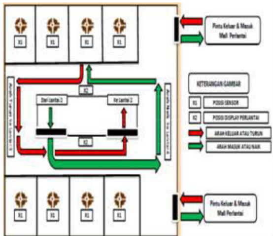
Gambar 3 Gambar Perancangan layout sistem parkir
