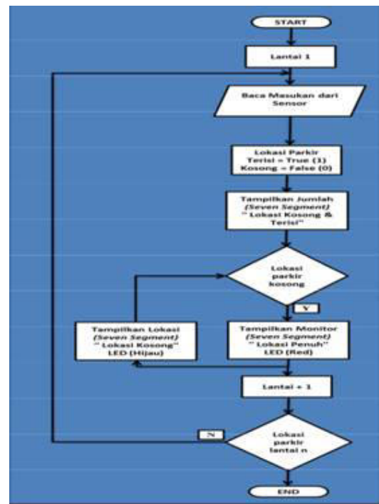
Gambar 9 Perancangan Flowchart Sistem
