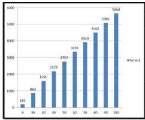
Gambar 13 Hasil Kurva Pembacaan Sensor Terhadap Jarak dan Waktu
