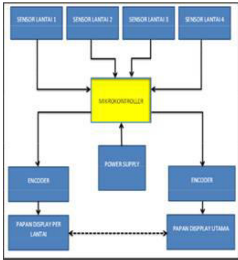
Gambar 1 Perancangan Block Diagram Sistem parkir otomatis berbasis mikrokontroler AVR Atmega 8535 dengan tampilan Seven Segment
