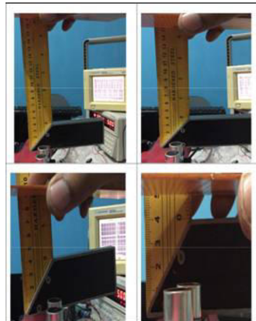
Gambar 12 Pengujian Mengukur Ketinggian Sensor Untuk Perlantai
