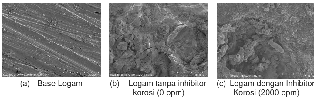
Gambar 3. Hasil pengujian SEM pada logam baja ASTM A36
