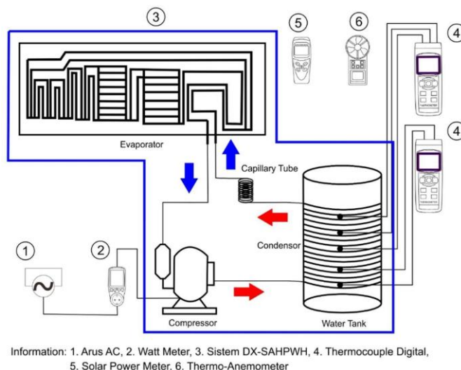
Gambar 3. Alat pemanas air dengan energi matahari dengan berbantuan pompa panas
