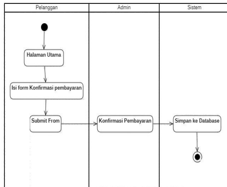
Gambar 9. Activity Diagram Konfirmasi
