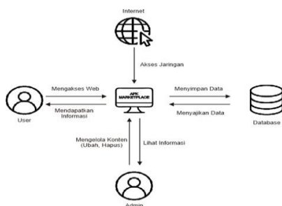
Gambar 2 Arsitektur Sistem
