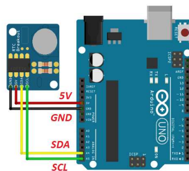
Gambar 1. Modul Arduino dan RTC
