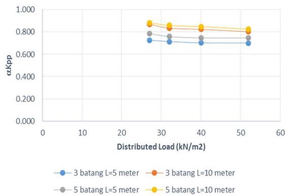
Gambar 16 \alpha_{Kpp} perkuatan cerucuk dan 1 lapis matras
