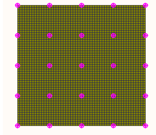
Gambar 5 Model perkuatan matras bambu pada Plaxis 3D Foundation 2.1 tampak atas
