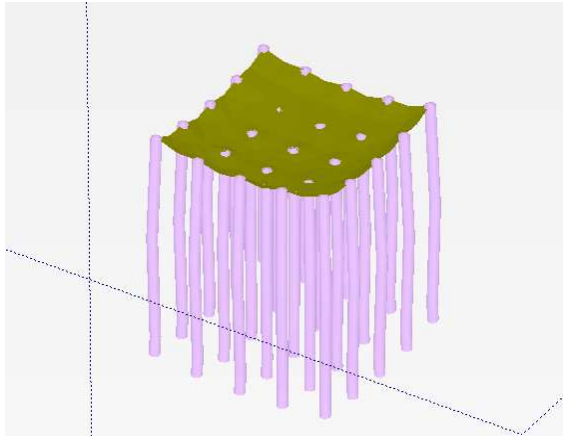
Gambar 7 Deformasi pada perkuatan cerucuk dan 1 lapis matras bambu
