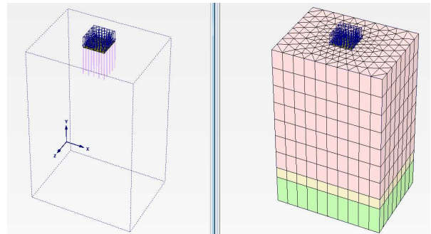
Gambar 6 Generated mesh 3D cerucuk dan 1 lapis matras bambu
