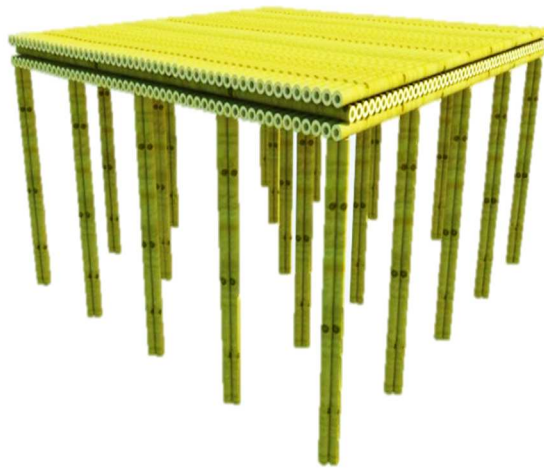
Gambar 3 Perkuatan Cerucuk dan 3 lapis matras bambu
