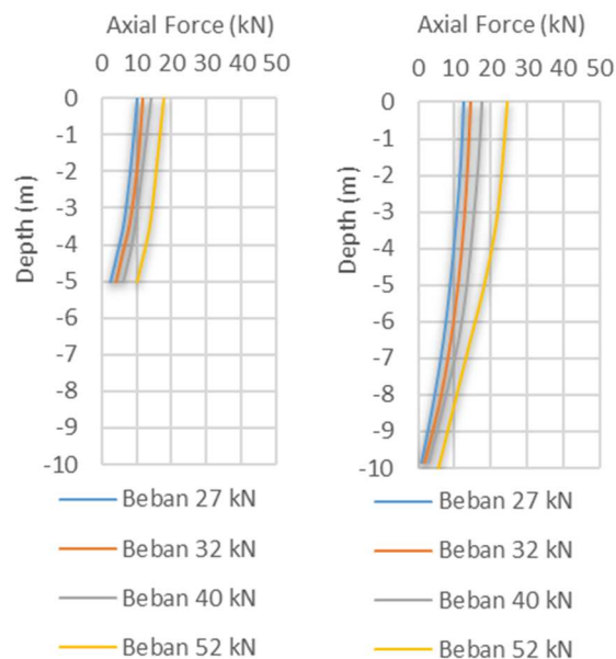
Gambar 15 Axial force pada 5 lapis matras & 3 batang cerucuk (panjang 5 dan 10 meter)
