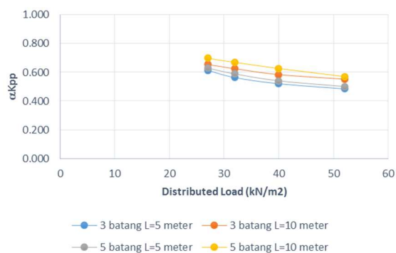
Gambar 18 \alpha_{Kpp} perkuatan cerucuk dan 3 lapis matras
