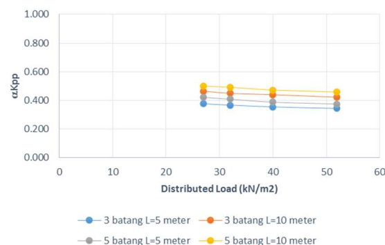
Gambar 19 \alpha_{Kpp} perkuatan cerucuk dan 5 lapis matras
