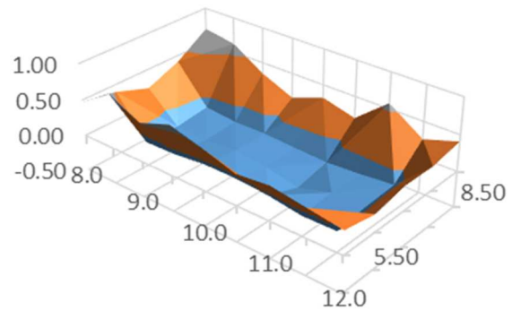
Gambar 7 Deformasi pada perkuatan cerucuk dan 1 lapis matras bambu
