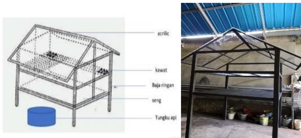
Gambar 2, Desain alat pengering hybrid dan alat pengeringan hybrid (Bidayani, et al, 2022)
