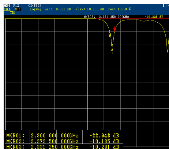
Gambar 11. Hasil pengujian return loss antenna MIMO 2x2
