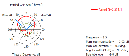
Gambar 8. Hasil simulasi pola radiasi elevasi antenna MIMO 2x2
