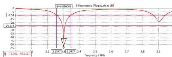
Gambar 5. Hasil simulasi bandwidth antenna MIMO 2x2
