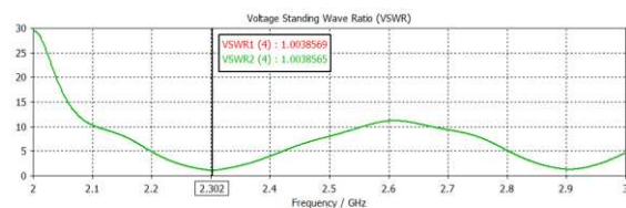
Gambar 4. Hasil simulasi VSWR antenna MIMO 2x2
