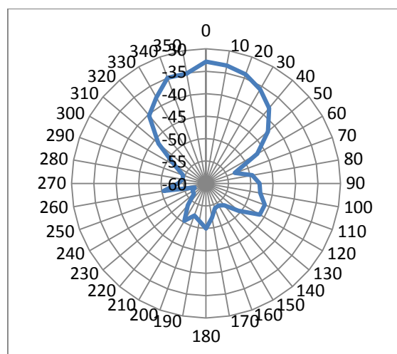
Gambar 16. Hasil pengujian pola radiasi elevasi antenna MIMO 2x2
