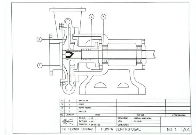
Gambar 2. Potongan Melintang Pompa Sentrifugal Hasil Rancangan Penelitian (Sumber: Penulis, 2025)
