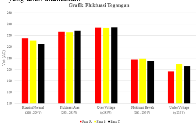
Gambar 7. Grafik Fluktuasi Tegangan
