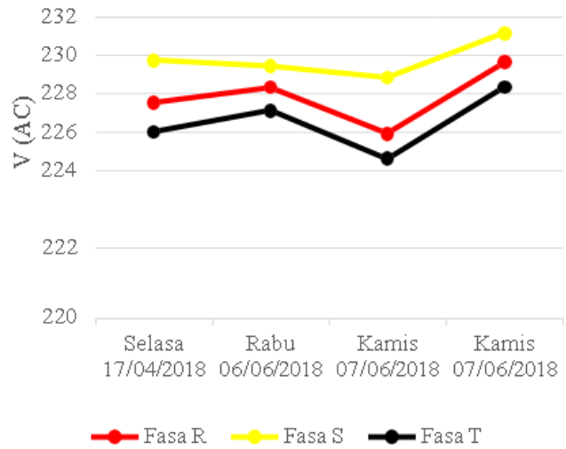
Gambar 5. Grafik Input Sensor Tegangan
