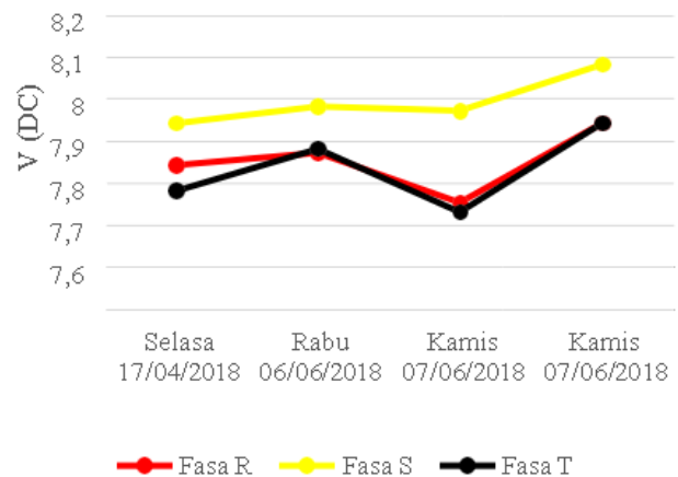
Gambar 6. Grafik Output Sensor Tegangan
