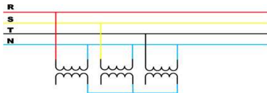
Gambar 4. Rangkaian Sensor Tegangan
