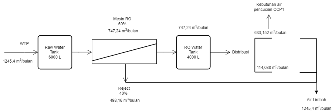
Gambar 3. Neraca Air Eksisting
