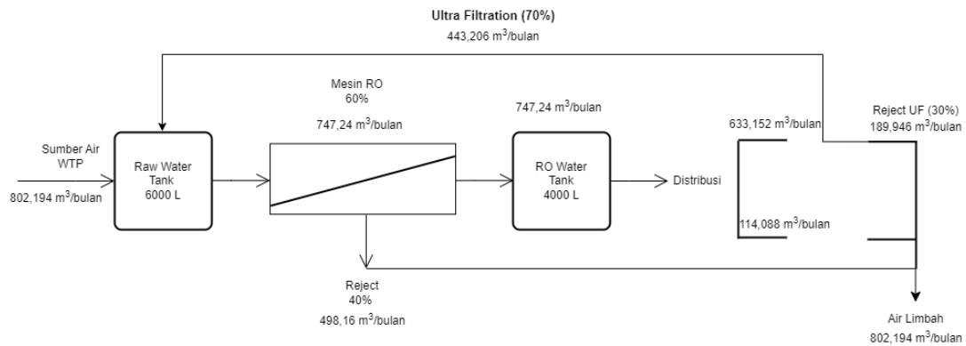
Gambar 5. Neraca Air Daur Ulang
