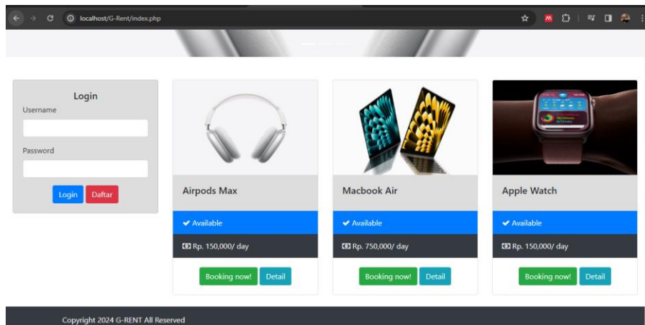
Gambar 1. 3 Halaman Login
