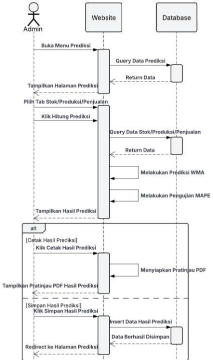
Gambar 5 Sequence Diagram Melakukan Prediksi
