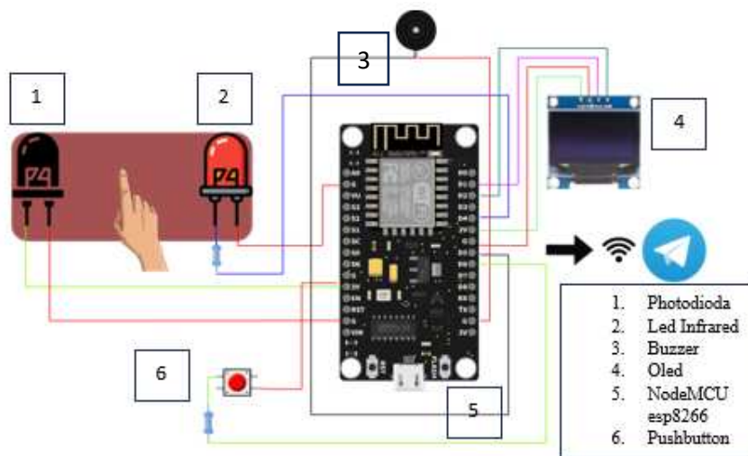
Gambar 2. Rancangan Sistem
