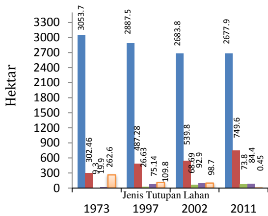
Gambar 3. Histogram luas tutupan lahan di zona inti.
