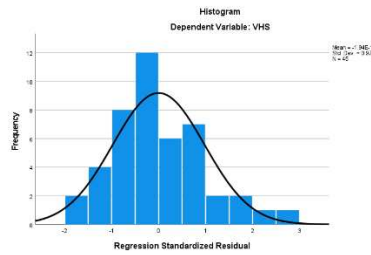
Gambar 1. Grafik Histogram Sumber: Output SPSS (2025)
