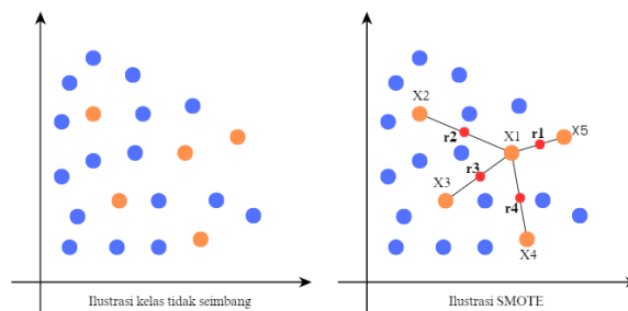
Gambar 2. Ilustrasi SMOTE
