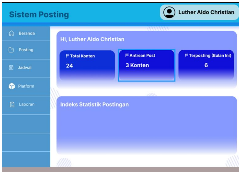
Gambar 6. Halaman Utama
