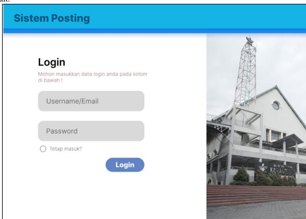
Gambar 5. Login Page
