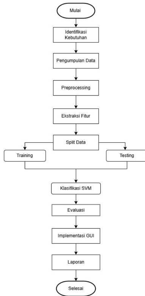
Gambar 1. Tahapan Penelitian
