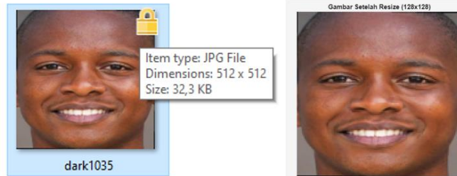
Gambar 3. Hasil Resize
