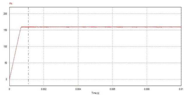
Gambar 19. Gelombang daya output pada intensitas cahaya 800 W/m².
