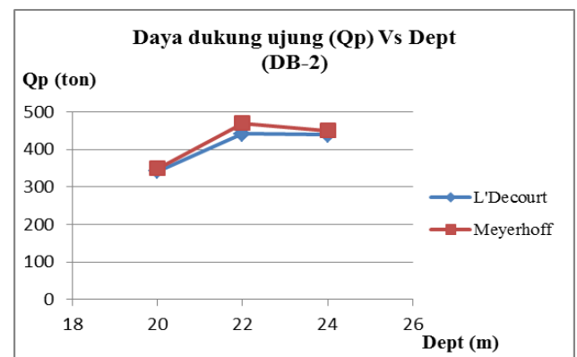
Gambar 7. Grafik Hasil Perhitungan Qp terhadap kedalaman pada DB2 (sumber: hasil perhitungan)
