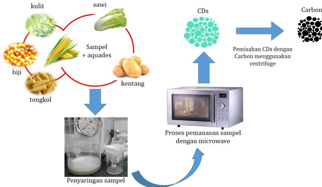
Gambar 1. Skema sintesis CDs dari bahan alam
