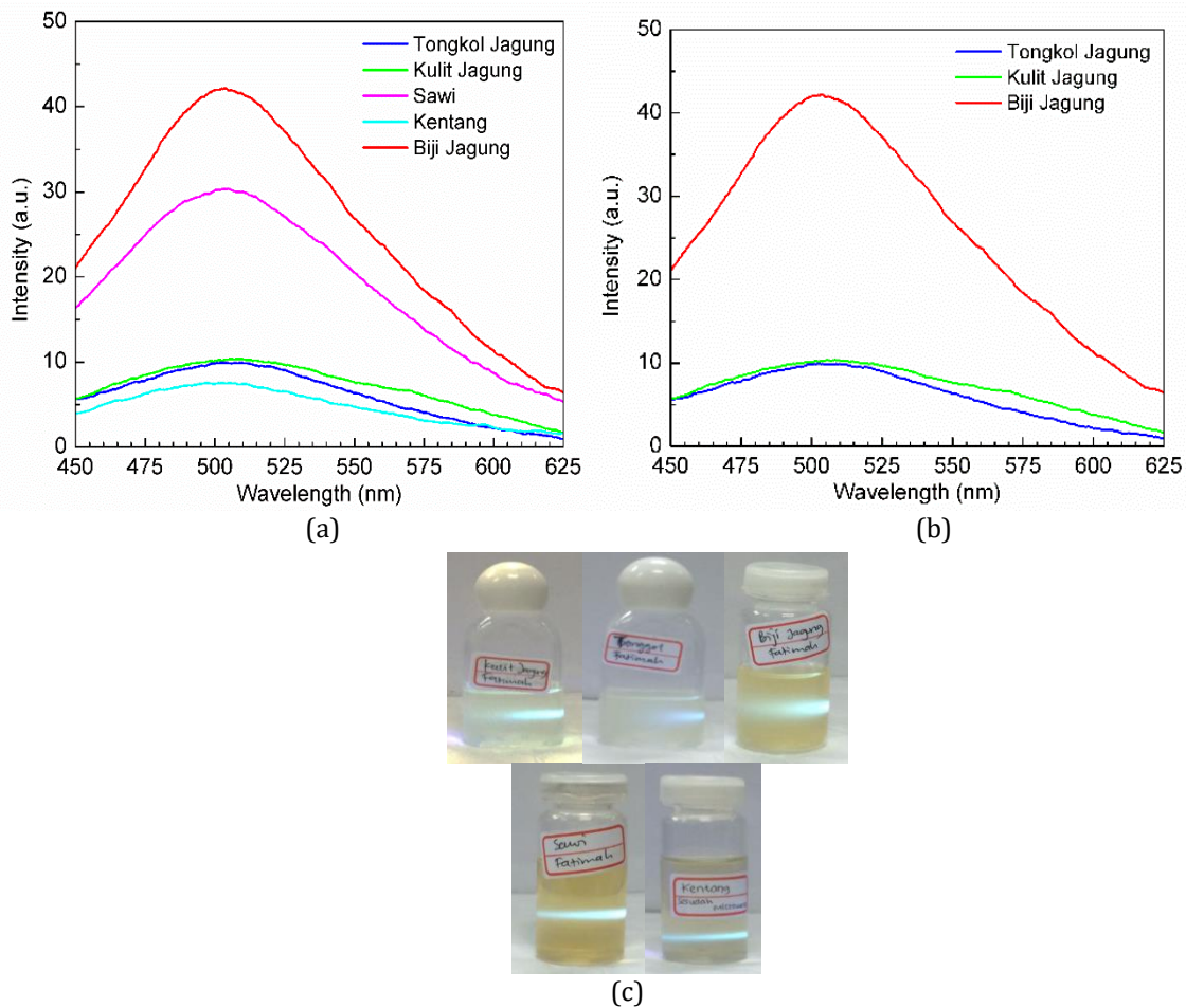
Gambar 3. (a) Grafik PL CDs bahan dan limbah organik, (b) Grafik PL CDs bagian-bagian jagung, (c) Pendaran sampel saat dieksitasi laser biru
