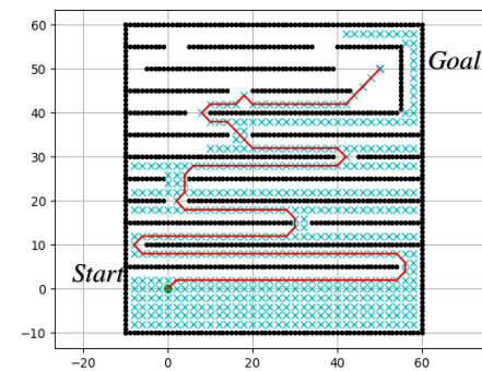
Gambar 11. Weighted A* pada Lingkungan pengujian narrow
