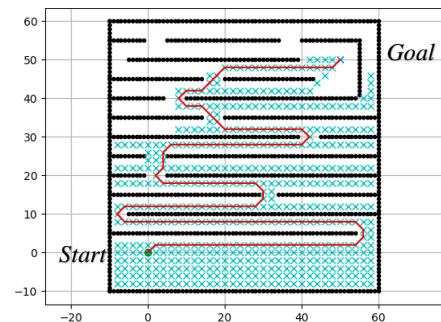
Gambar 10. A* pada Lingkungan pengujian narrow
