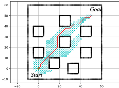
Gambar 6. A* pada Lingkungan pengujian clutter
