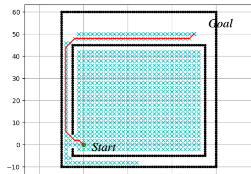
Gambar 12. A* pada Lingkungan pengujian trap
