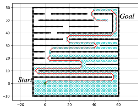
Gambar 16. Weighted A* pada lingkungan narrow
