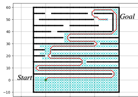
Gambar 15. Weighted A* pada lingkungan narrow
